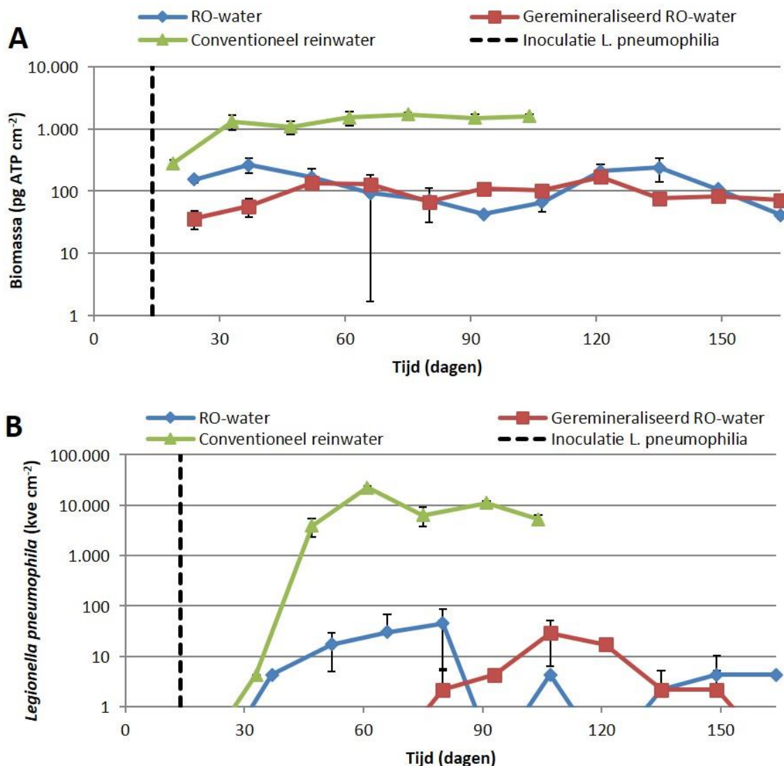
Afbeelding 1. A) De ATP-concentratie en B) het aantal kolonievormende eenheden (kve) L. pneumophila op de glazen ringen uit de BBM, gevoed met de drie verschillende watertypes: conventioneel reinwater (groen), RO-water (blauw) en geremineraliseerd RO-water (rood)
