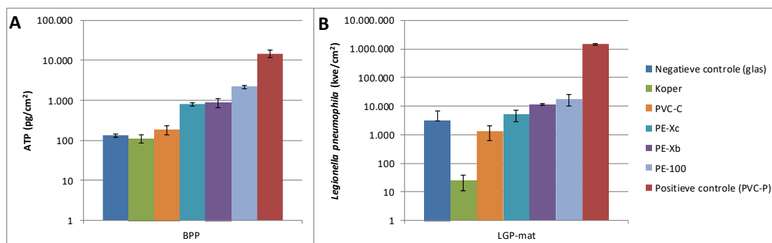
Afbeelding 3. A) De biomassaproductiepotentie (BPP) en (B) de legionellagroeiopotentie (LGP) van de onderzochte leidingmaterialen in contact met geremineraliseerd RO-water
