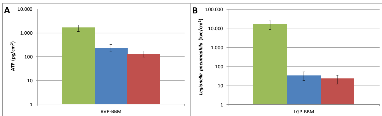
Afbeelding 2. A) De biofilmvormingsspotentie (BVP) en de legionellagroeiopotentie (LGP) van conventioneel drinkwater (groen), RO-water (blauw) en geremineraliseerd RO-water (rood) bepaald met de BBM
